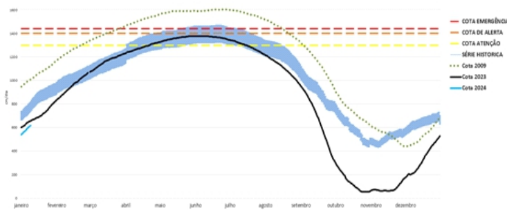
COTAGRAMA 2: RIO NEGRO - MANAUS ESTÇÃO - 14990000 Maior cheia em 18/06/2021, com cota de 1922 cm.
