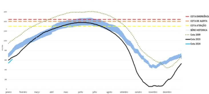
COTAGRAMA 1: RIO AMAZONAS - ITACOATIARA ESTÇÃO - 16090000
