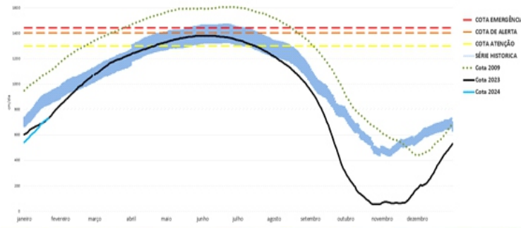
COTAGRAMA 2: RIO NEGRO - MANAUS ESTÇÃO - 14990000 Maior cheia em 20/06/2021, com cota de 2085 cm.
