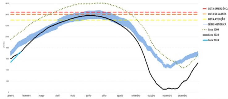
COTAGRAMA 2: RIO NEGRO - MANAUS ESTÇÃO - 14990000 Maior cheia em 18/06/2021, com cota de 1682 cm.
