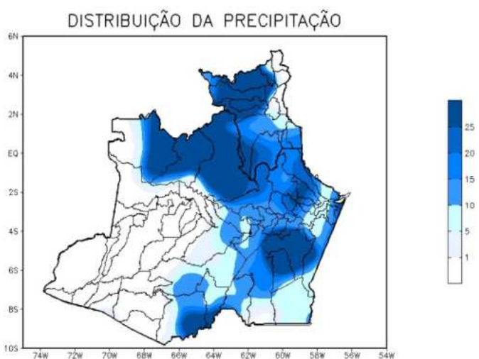
Figura 3: Mapa de distribuição da precipitação no estado do Amazonas e Roraima no dia 15/02/2022
