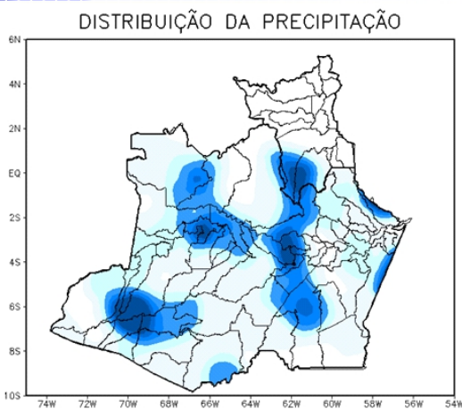
Figura 3: Mapa de distribuição da precipitação no estado do Amazonas e Roraima no dia 10/04/2023
