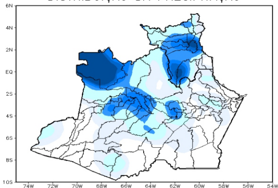
Figura 3: Mapa de distribuição da precipitação no estado do Amazonas e Roraima no dia 09/06/2023
