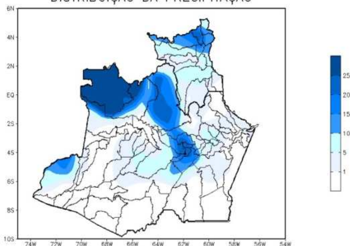
Figura 3: Mapa de distribuição da precipitação no estado do Amazonas e Roraima no dia 21/06/2022
