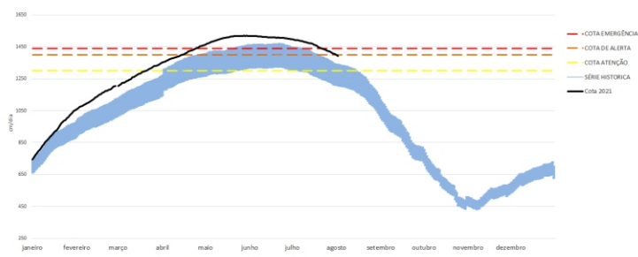
COTAGRAMA 2: RIO NEGRO - MANAUS ESTAÇÃO - 14910000
