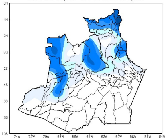
Figura 3: Mapa de distribuição da precipitação no estado do Amazonas e Roraima no dia 27/07/2022
