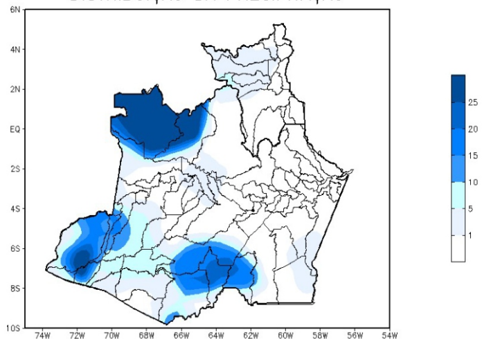
Figura 3: Mapa de distribuição da precipitação no estado do Amazonas e Roraima no dia 05/08/2022
