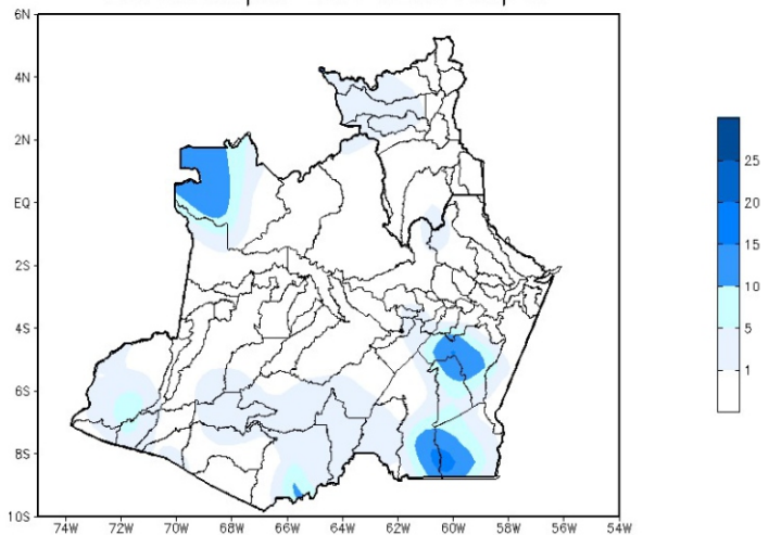
Figura 3: Mapa de distribuição da precipitação no estado do Amazonas e Roraima no dia 10/08/2022
