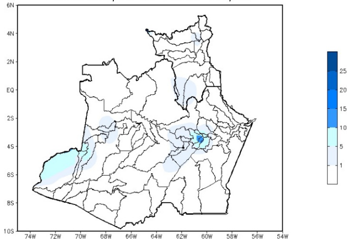
Figura 3: Mapa de distribuição da precipitação no estado do Amazonas e Roraima no dia 16/08/2022
