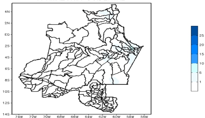
Figura 3: Mapa de distribuição da precipitação no estado do Amazonas e Roraima no dia 17/08/2023
