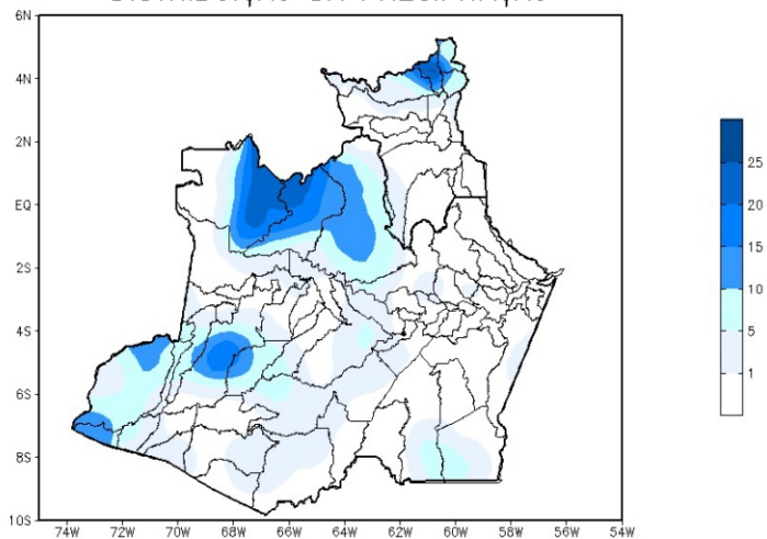
Figura 3: Mapa de distribuição da precipitação no estado do Amazonas e Roraima no dia 30/08/2022
