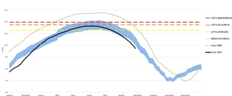
COTAGRAMA 1: RIO AMAZONAS - ITACOATIARA ESTÇÃO - 16030000
