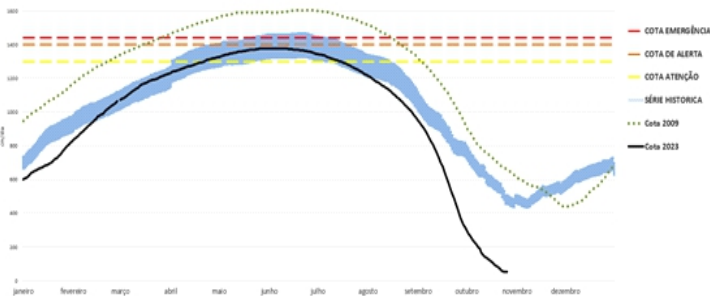
COTAGRAMA 2: RIO NEGRO - MANAUS ESTÇÃO - 14990000 Maior cheia em 24/06/2021, com cota de 1969 cm.
