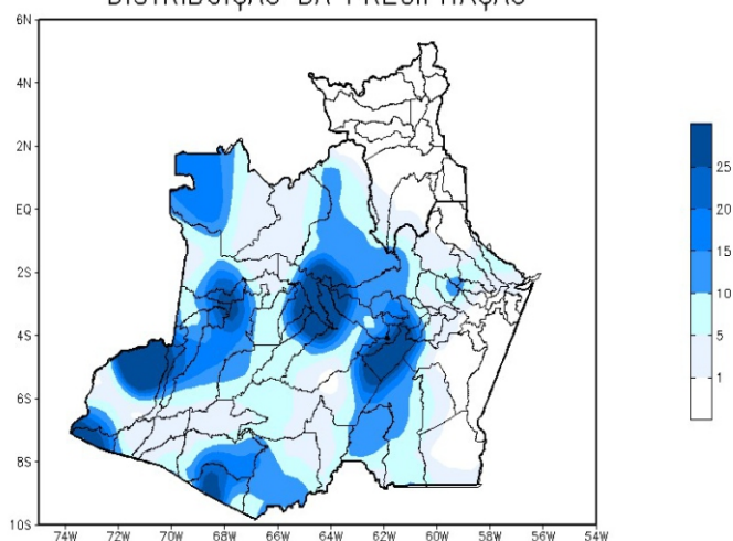
Figura 3: Mapa de distribuição da precipitação no estado do Amazonas e Roraima no dia 30/12/2021
