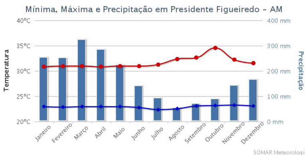
ILUSTRAÇÃO 2.3.3: DADOS CLIMATOLÓGICOS: MÉDIA DO PERÍODO ENTRE 1961 E 1990 EM PRESIDENTE FIGUEIREDO. (FONTE: JORNAL DO TEMPO)
