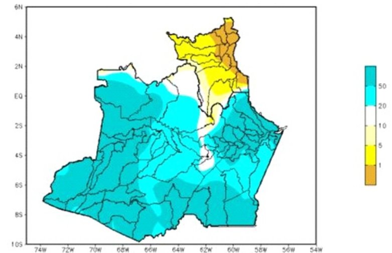
Figura 2: Mapa de Distribuição de Precipitação no Amazonas do período de 07 a 13/01/2018
