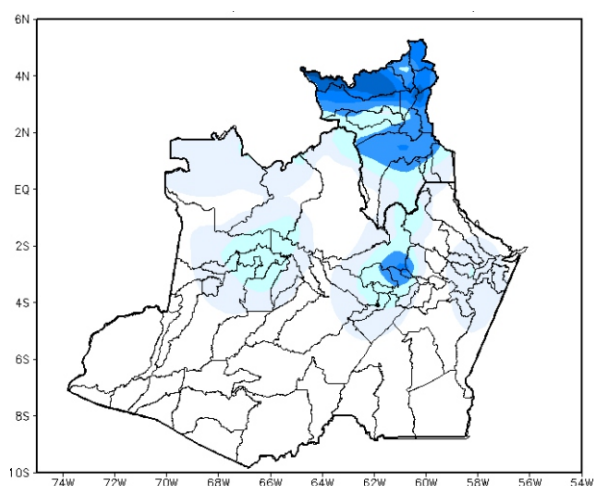
Figura 3: Mapa de distribuição da precipitação no estado do Amazonas no dia 23/07/2020
