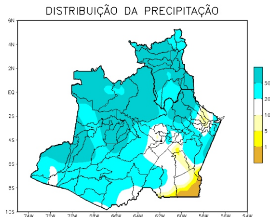
Figura 2 - mapa de distribuição de precipitação no Amazonas do período de 07 a 13/05/2018
