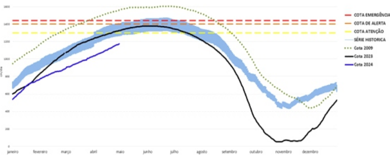
COTAGRAMA 2: RIO NEGRO - MANAUS ESTÇÃO - 14990000 Maior cheia em 14/07/2023, com cota de 2561 cm.
