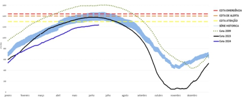
COTAGRAMA 2: RIO NEGRO - MANAUS ESTÇÃO - 14990000 Maior cheia em 16/06/2021, com cota de 2994 cm.
