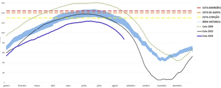
COTAGRAMA 2: RIO NEGRO - MANAUS ESTÇÃO - 14990000 Maior cheia em 24/06/2021, com cota de 2677 cm.
