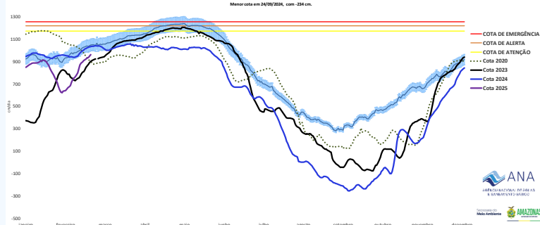
COTAGRAMA - TABATINGA ESTAÇÃO - 10100000 Maior cota em 20/05/2021, com 13,82 cm. Menor cota em 24/09/2024, com -254 cm.
