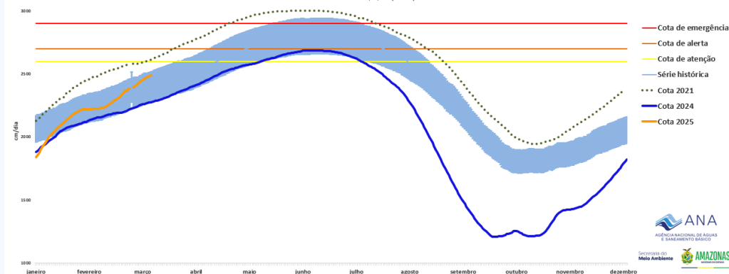
COTAGRAMA 2: RIO NEGRO - MANAUS ESTÇÃO - 14990000 Maior cota em 16/04/2021, com 30,02 cm. Menor cota em 12/10/2024, com 12,11 cm.
