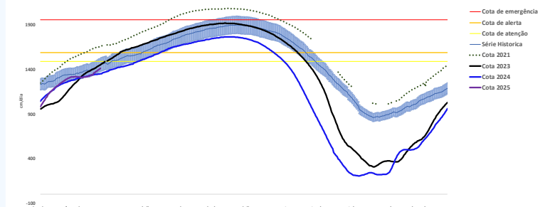
COTAGRAMA - MANACAPURU ESTÇÃO - 10100000 Maior cota em 18/06/2021 com cota de 20,86 cm
