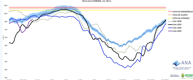
COTAGRAMA - TABATINGA ESTÇÃO - 10100000 Maior cota em 23/05/2020, com 12,82 cm. Menor cota em 24/06/2024, com -254 cm.
